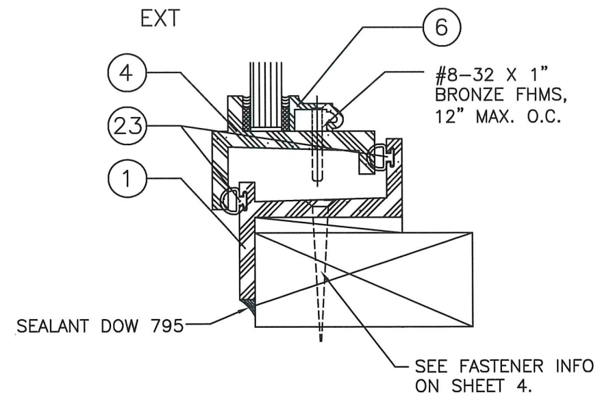
(D) SILL
