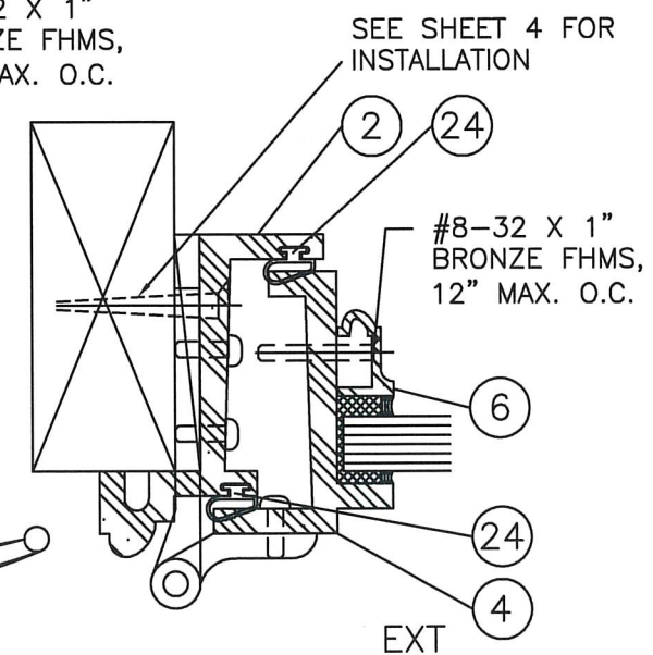
(F) JAMB
